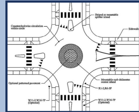
MINI ROUNDABOUT
